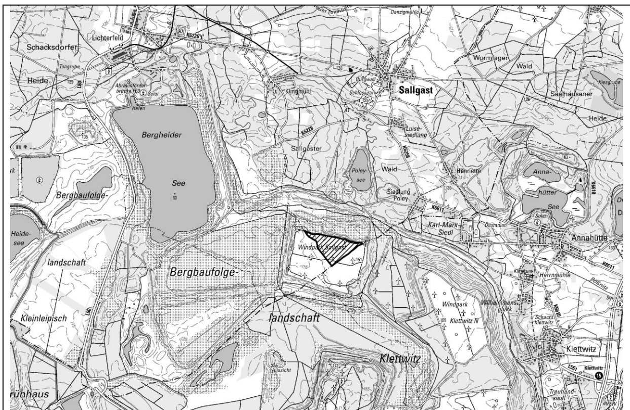
Geltungsbereich des Bebauungsplans „Sondergebiet Energiestandort Hochkippe für den Bereich Sallgast“
